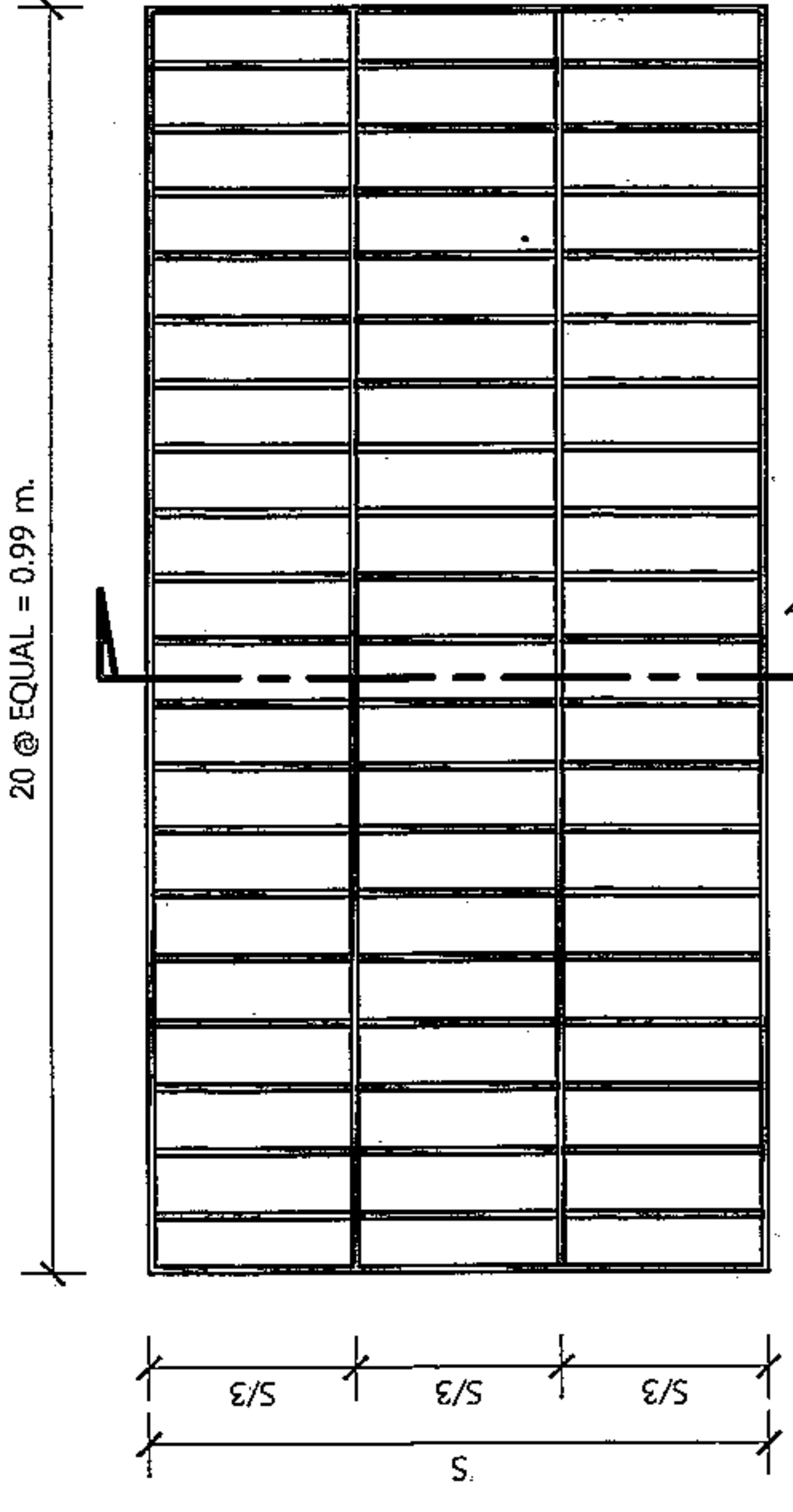
FLAT BAR 44 x 9 mm. เชื่อมตลอดแนวรอยต่อทุกด้าน
