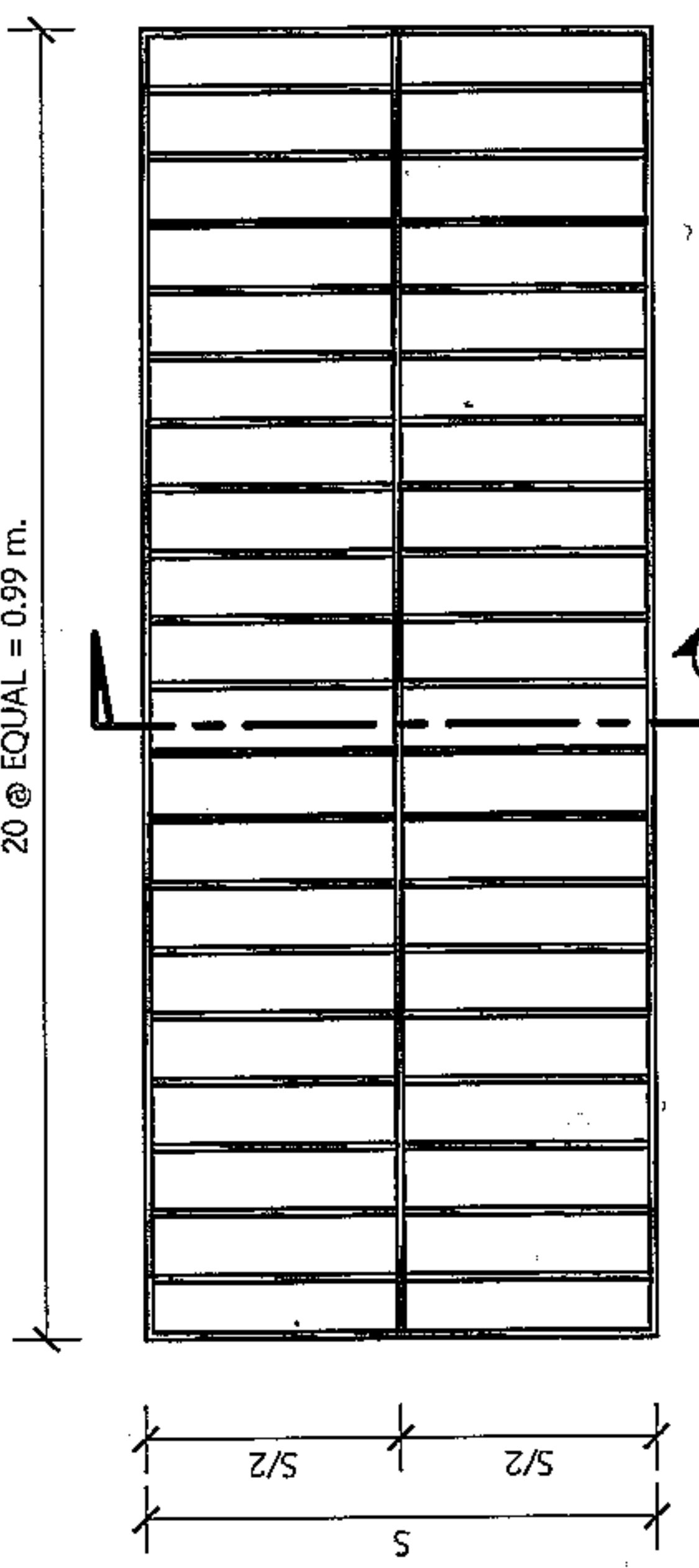
FLAT BAR 44 x 9 mm. เชื่อมตลอดแนวรอยต่อทุกด้าน
