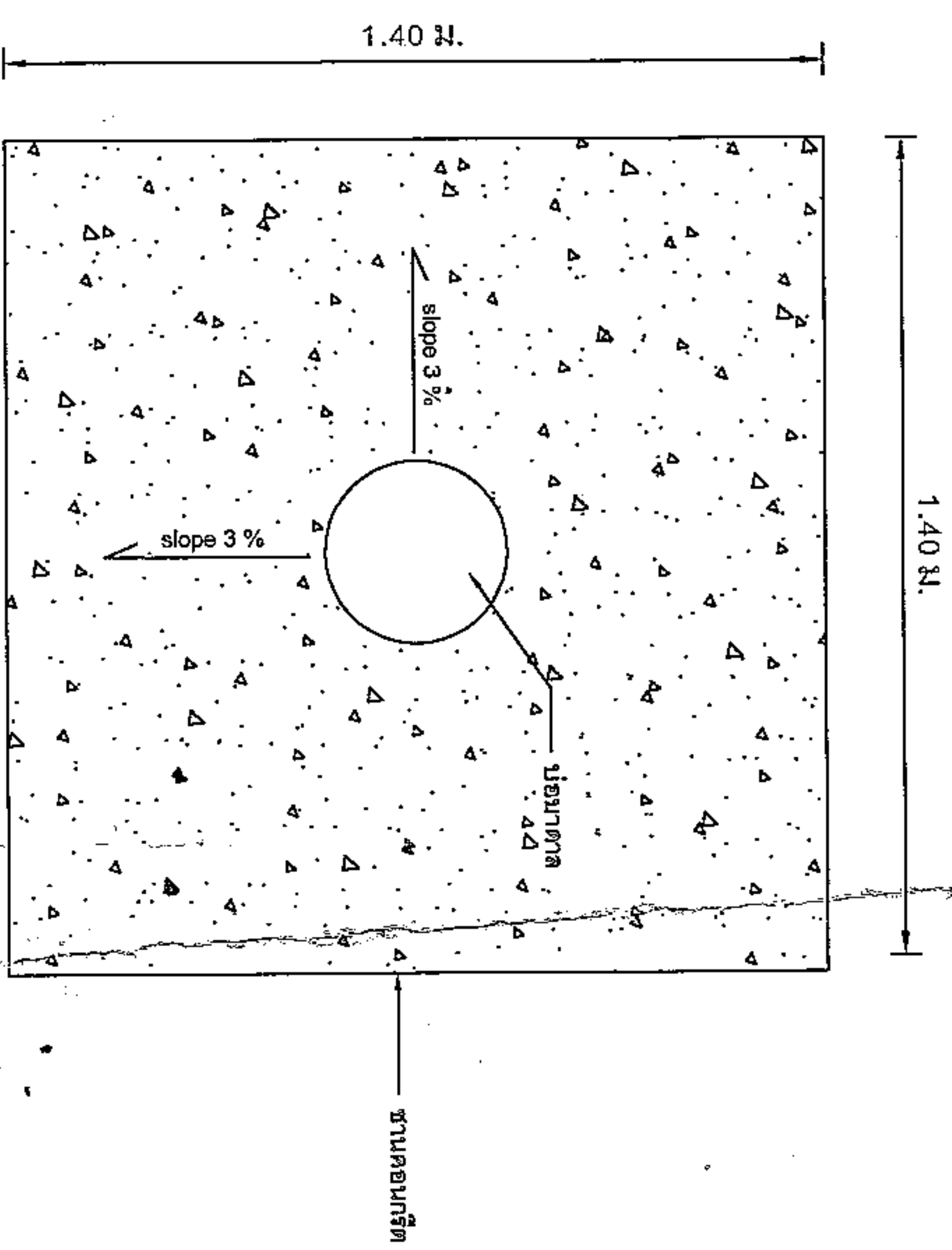
แบบฐานบ่อน้ำบาดาล SCALE Not to Scale
