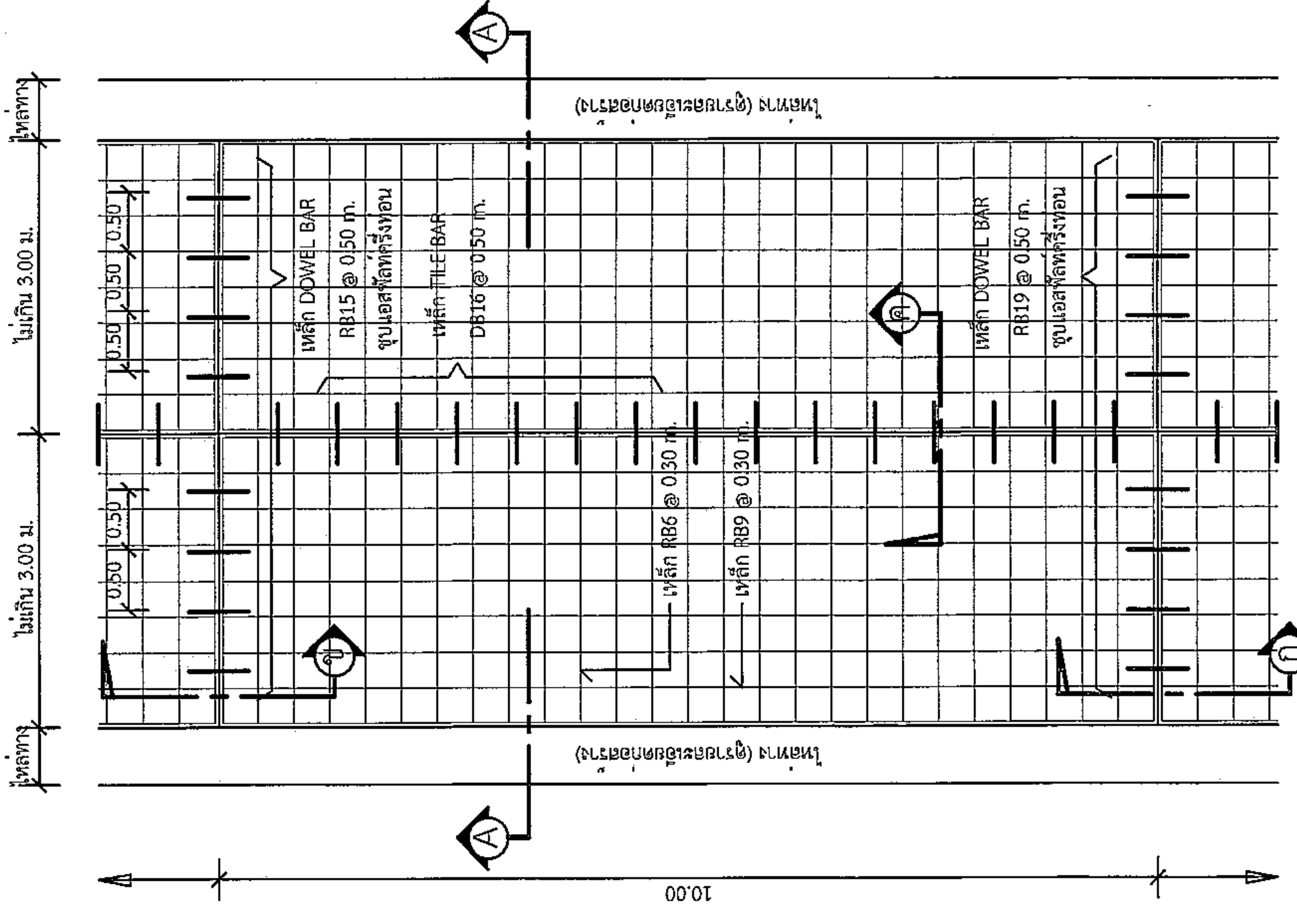
แปลนพื้นถนน 1 : 75
